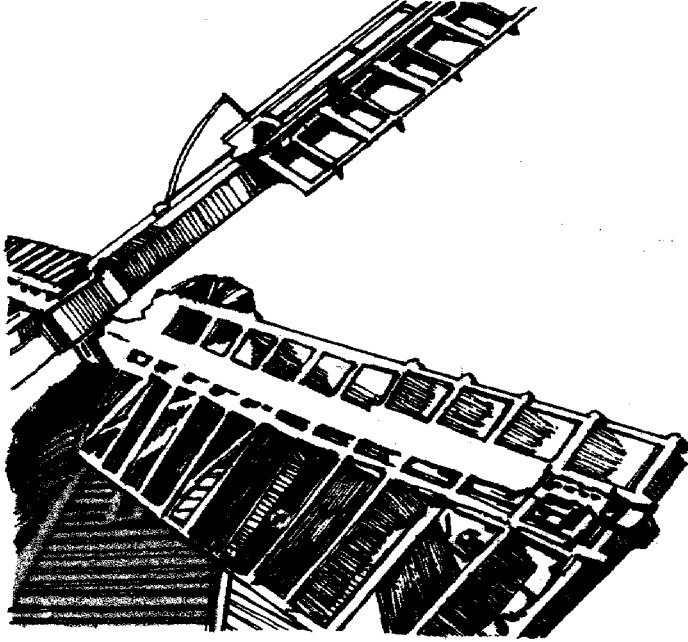
चित्र 11. सैंडविच, केंट में कप्तानीदार पालों का एक निकट का दृश्य। वायु के झोंके के अचानक आने पर स्प्रिंग का दबाव शर्ट्स को खोल देता है, जिससे वायु आराम से बाहर निकल जाती है।
